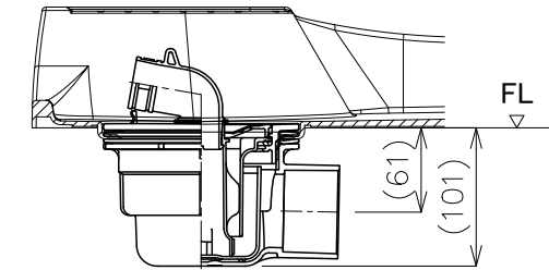
設置例: 横引排水トラップ 【有色】SCT-SNW、【透明】SCT-C-SNW
