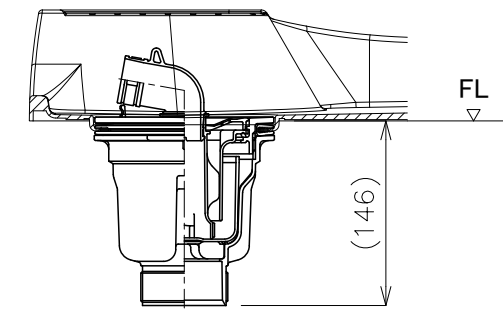
設置例: 縦引排水トラップ 【有色】SYT-SNW
