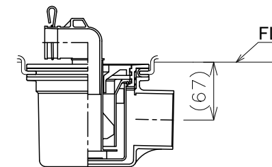
設置例: 横引排水トラップ【透明】CT-SNW/W
