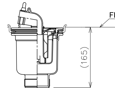
設置例: 縦引排水トラップ【有色】YT-SNW/W
