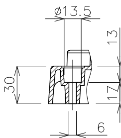
断面 B-B (詳細図 S=1:3)
