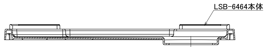
断面 A-A
