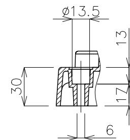
断面 B-B (詳細図 S=1:3)
