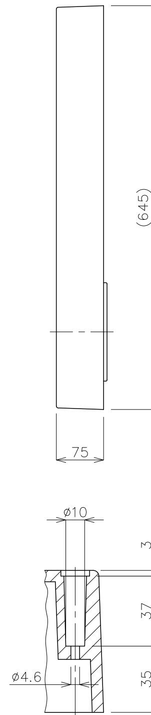
断面 B-B(S=1:2)
