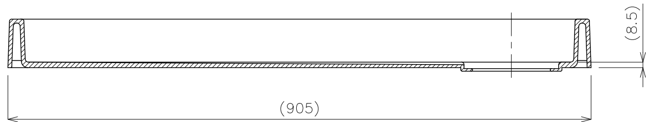
断面 A-A
