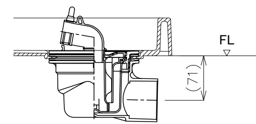
設置例: 横引排水トラップ 【有色】XT-SNW、【透明】XT-C-SNW
