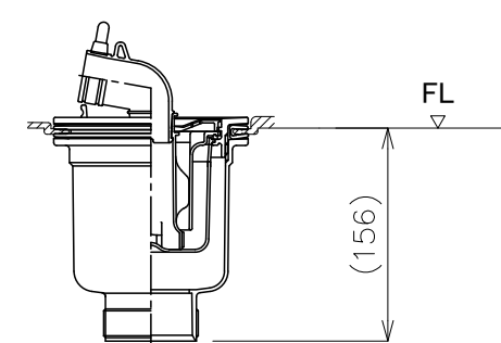
設置例: 縦引排水トラップ 【有色】YT-SNW
