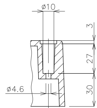
断面 B-B(S=1:2)
