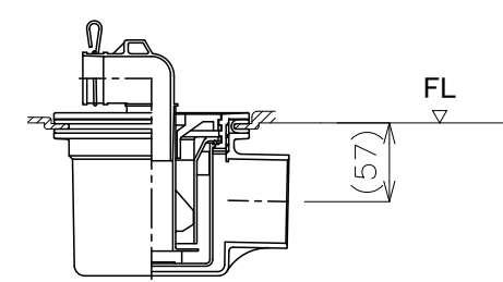
設置例: 横引排水トラップ 【透明】CT-SNW
